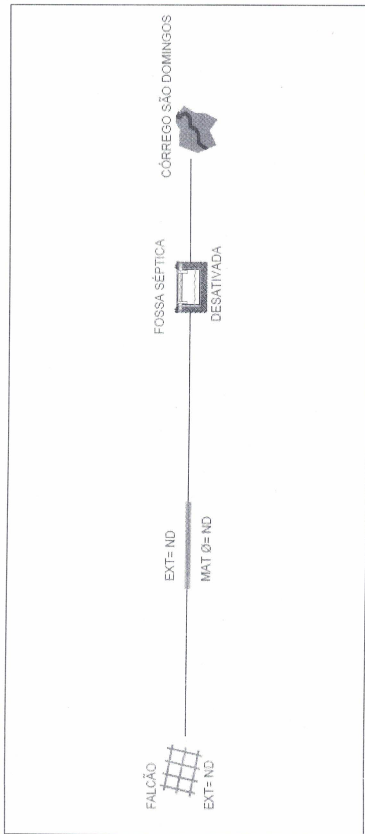
Figura 25 – Esquema do SES do distrito de Falcão
